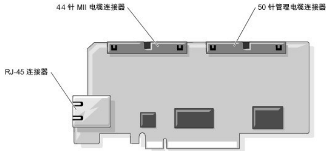
图 1-1. DRAC 5 硬件配置
