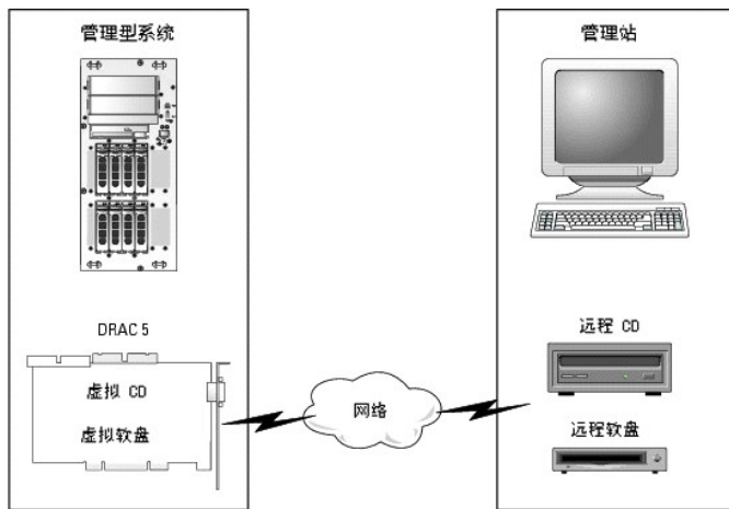
图 8-1. 虚拟介质的整体系统结构
